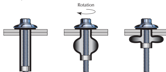
Figure 1 - Mise en oeuvre de la vis en aveugle
